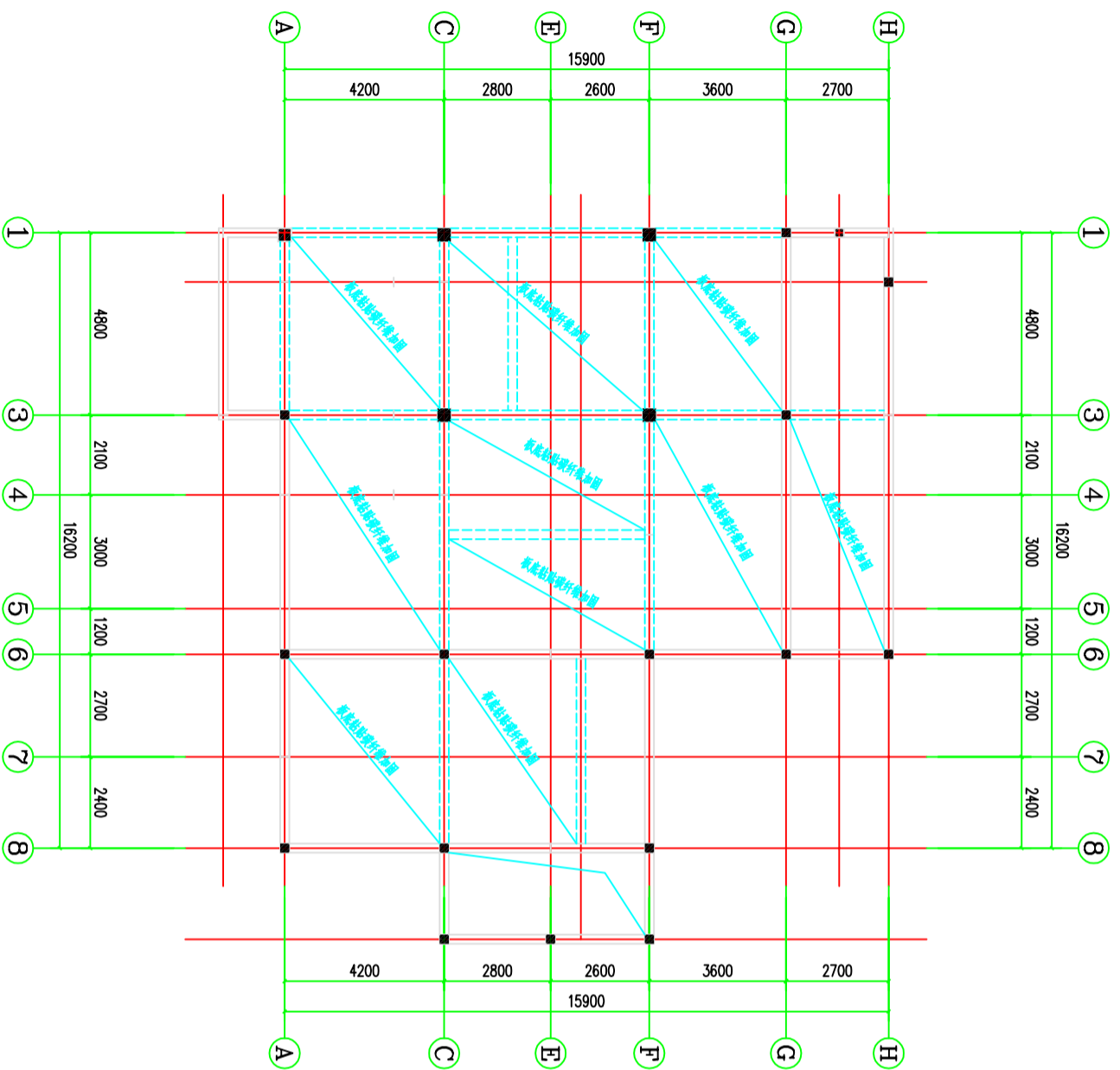
四层顶加固布置图
